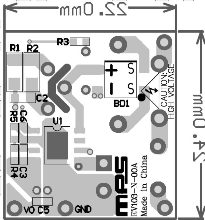
Figure 4 — Bottom Layer
